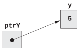
Figura 7.2 Representación gráfica de un apuntador que apunta hacia una variable entera en memoria.
