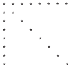
Figura 6.26 Los 22 cuadros eliminados al colocar una reina en la esquina superior izquierda.
