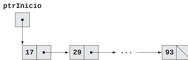
Figura 12.2 Representación gráfica de una lista ligada.
