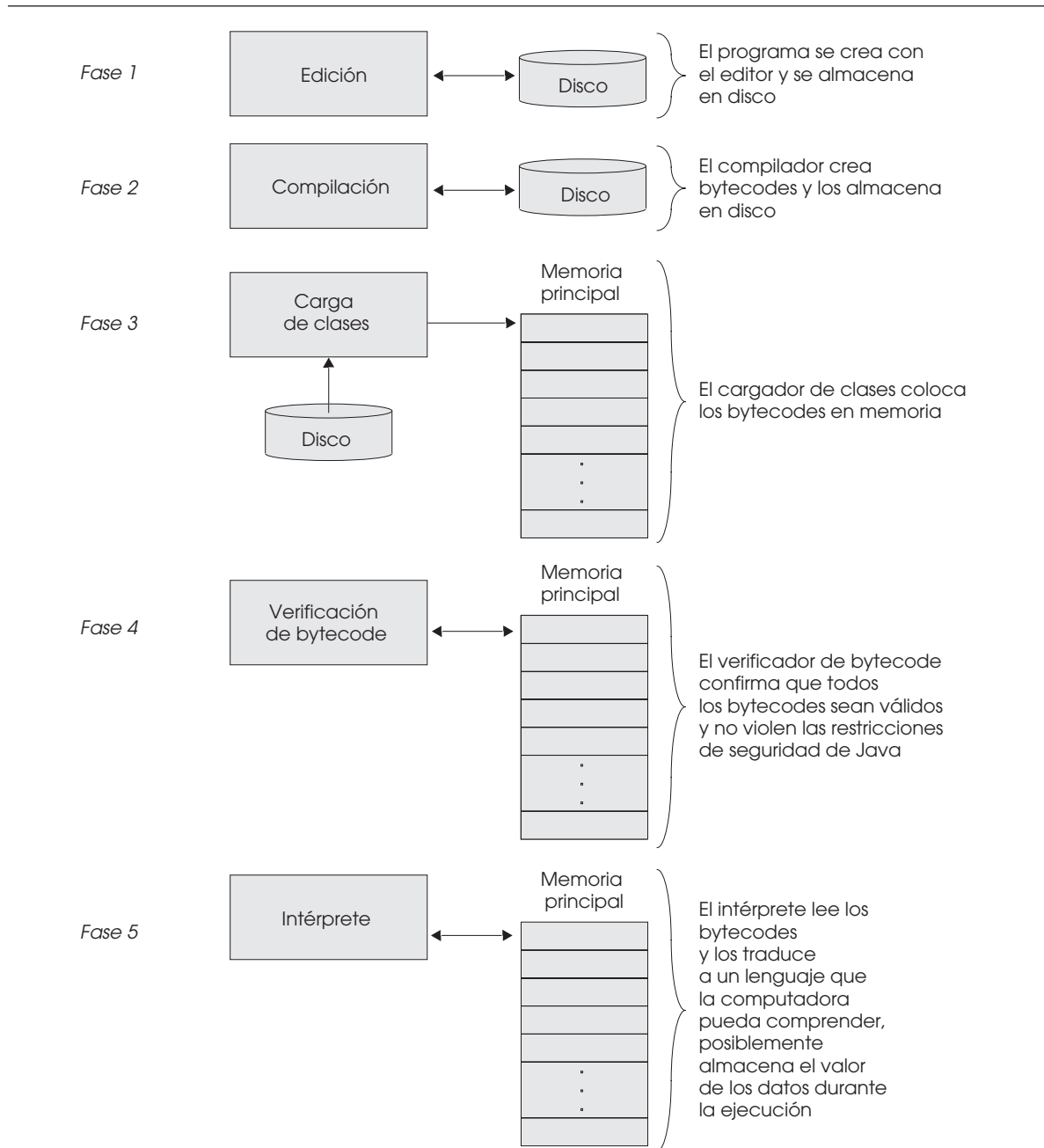
Figura 24.1 Un típico ambiente de Java.
