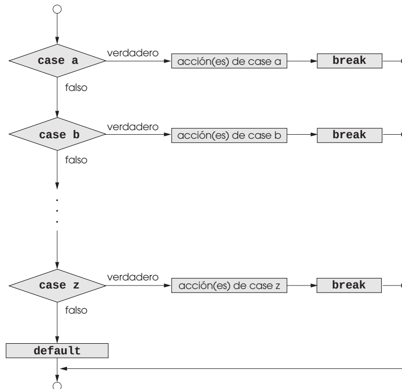
Figura 4.8 Instrucción de selección múltiple switch con breaks .
